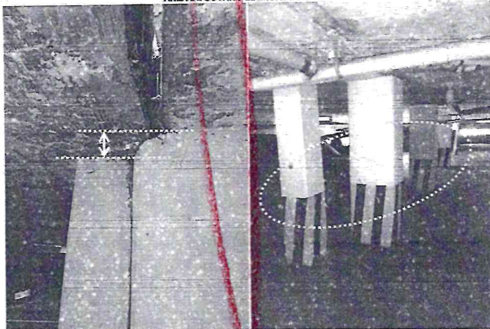
Se observan fisuras diagonales en la parte central de columnas, así como emersión diferencial.
