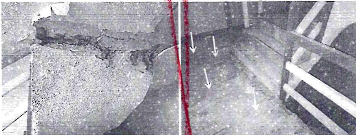
En todos los arranques y uniones de la escalera se aprecian con desconchamiento y exposición del acero.
