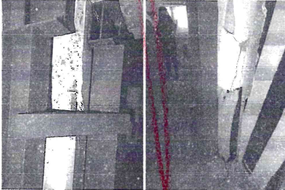
Columnas dañadas (fracturas diagonales, desconchamiento y exposición del acero de refuerzo) con apuntalamientos metálicos precarios de baja calidad en materiales y calidad técnica.
