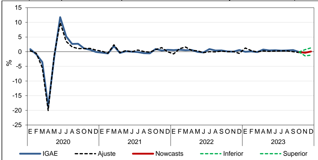
Gráfica 4 IOAE: NOWCAST DEL IGAE MODELOS ESTIMADOS CON SERIES DESESTACIONALIZADAS (variación porcentual real respecto al mes anterior: noviembre y diciembre de 2023)
