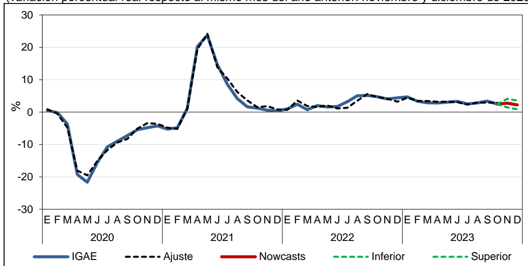
Gráfica 3 IOAE: NOWCAST DE LAS ACTIVIDADES TERCIARIAS MODELOS ESTIMADOS CON SERIES DESESTACIONALIZADAS (variación porcentual real respecto al mismo mes del año anterior: noviembre y diciembre de 2023)
