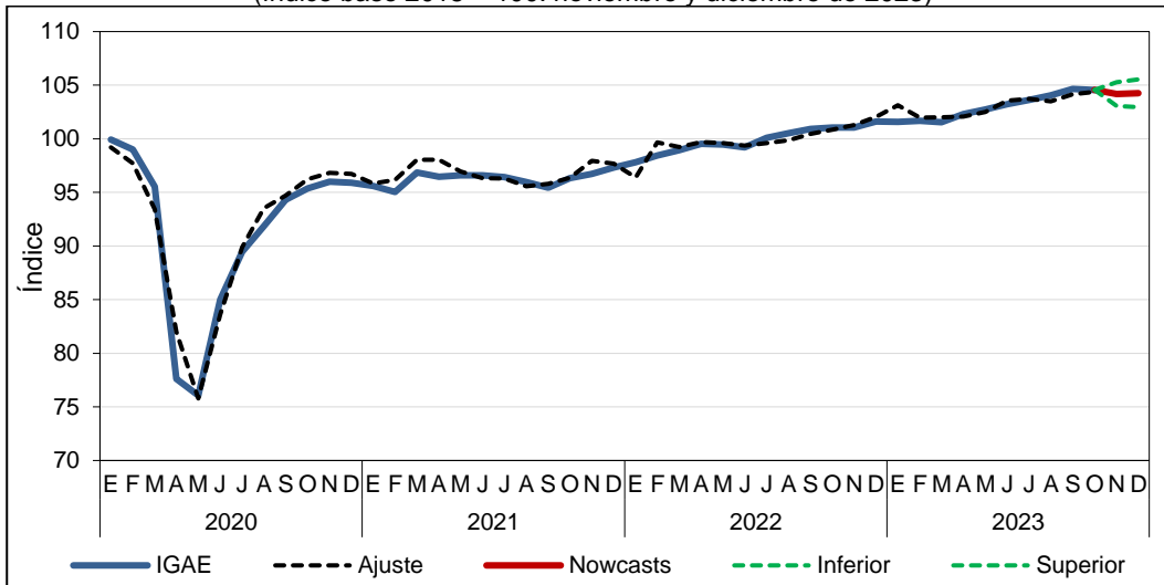
Gráfica 5 IOAE: NOWCAST DEL IGAE MODELOS ESTIMADOS CON SERIES DESESTACIONALIZADAS (índice base 2018 = 100: noviembre y diciembre de 2023)
